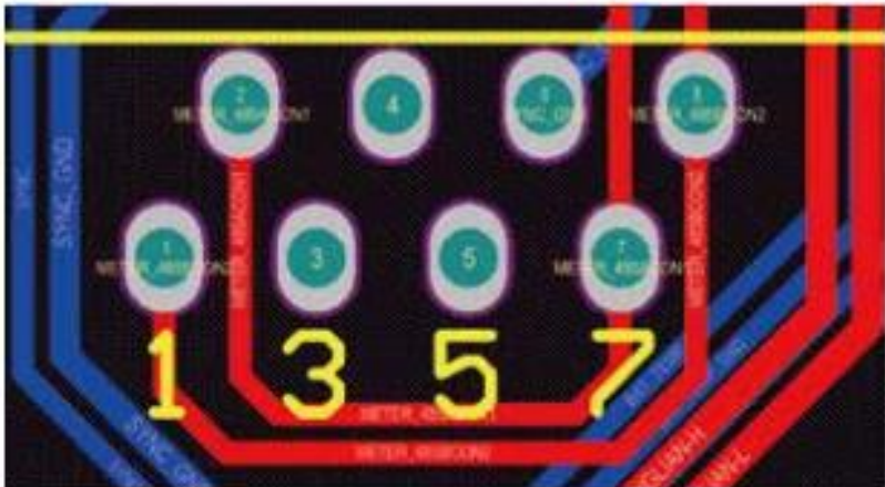
RS-485 Port
